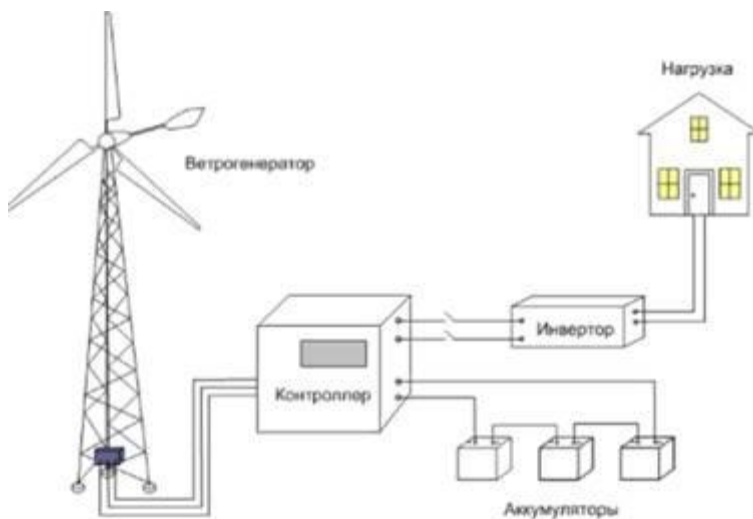
Рисунок. 2. Работа ветрогенератора
